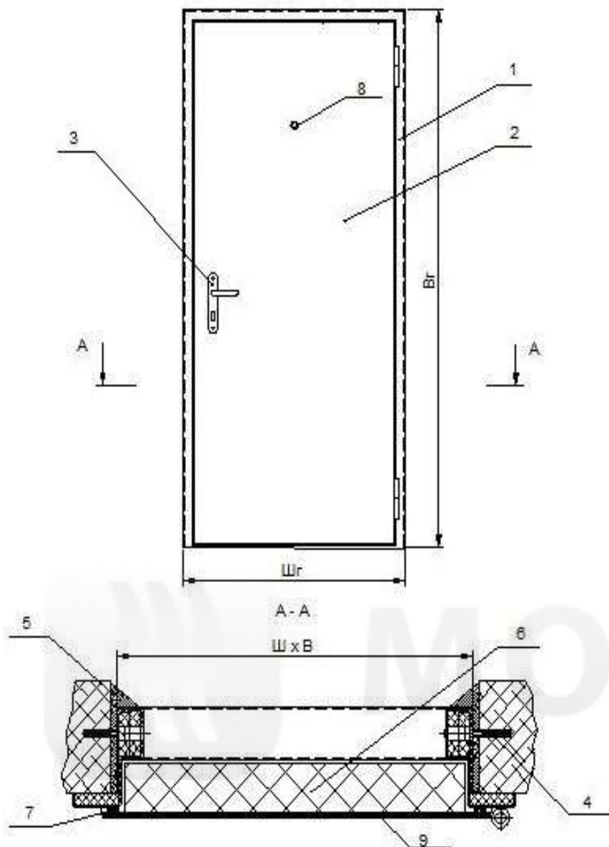
Рис. 1 Общий вид дверей ДМ-х, МД-х, ДМУ-1, ДМУ-2
